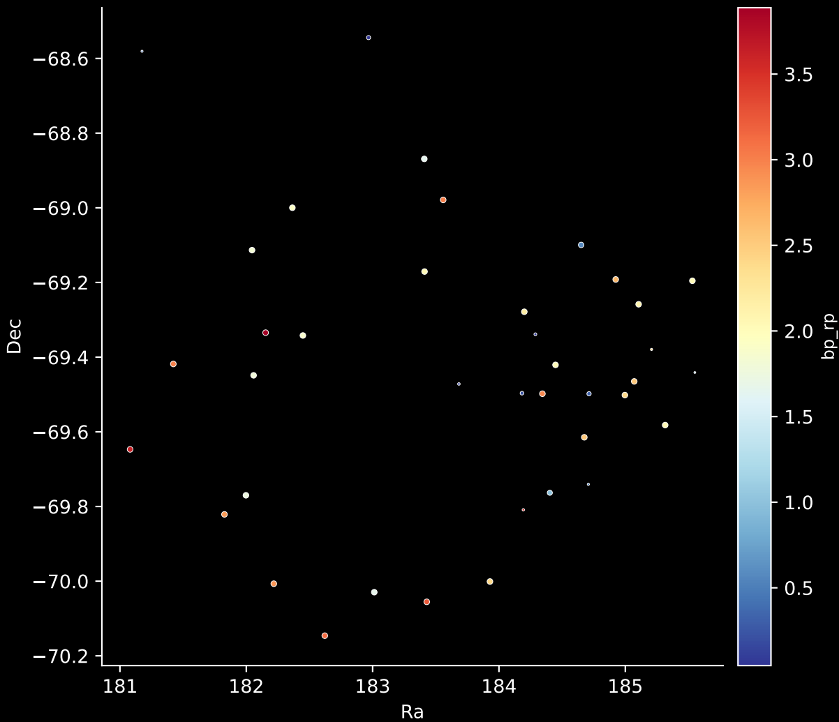
APOGEE DR17 Field: [280-32-O] Stars: 39
