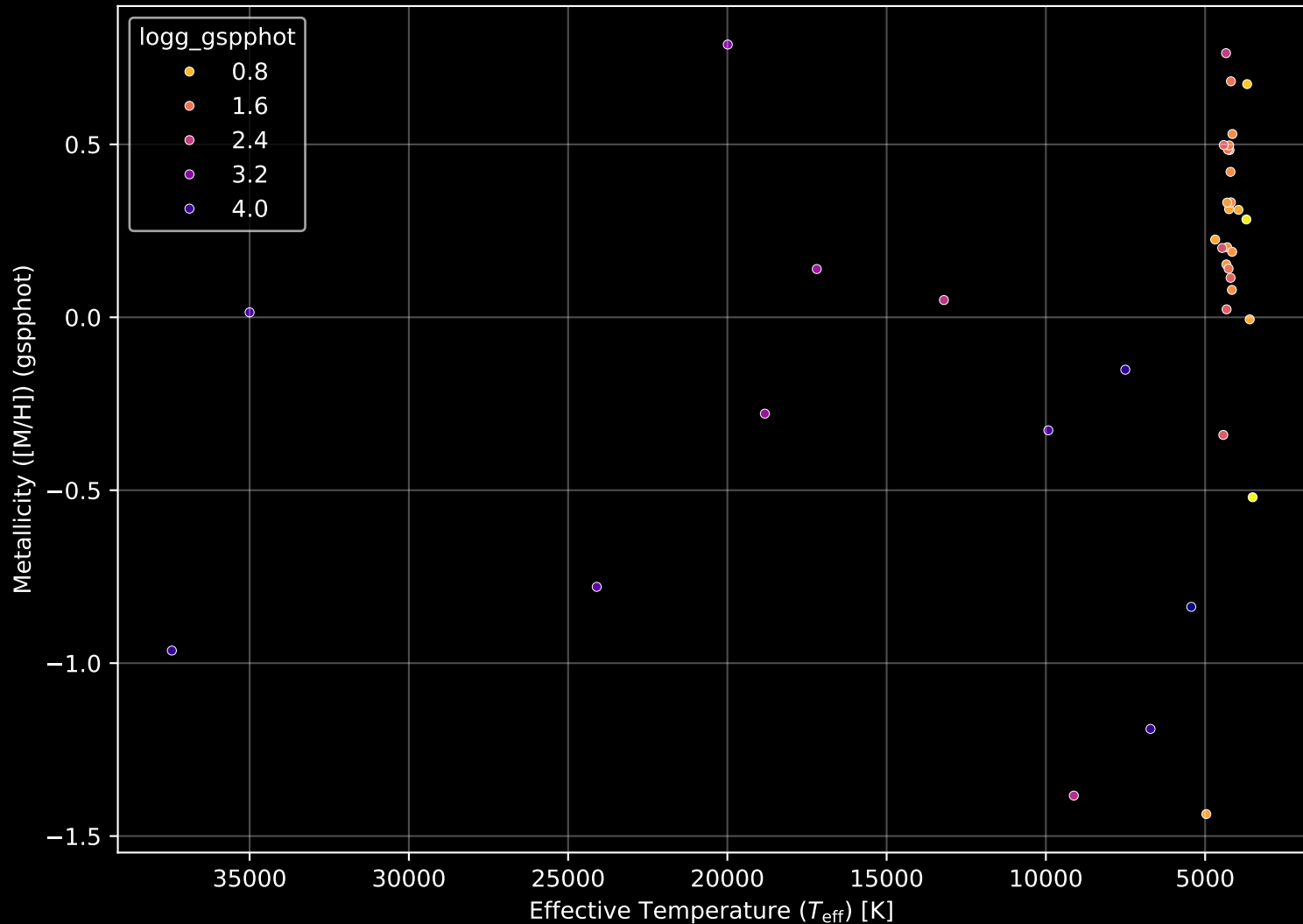
APOGEE DR17 Field: [280-32-O] Stellar Population Parameters (n= 39)
