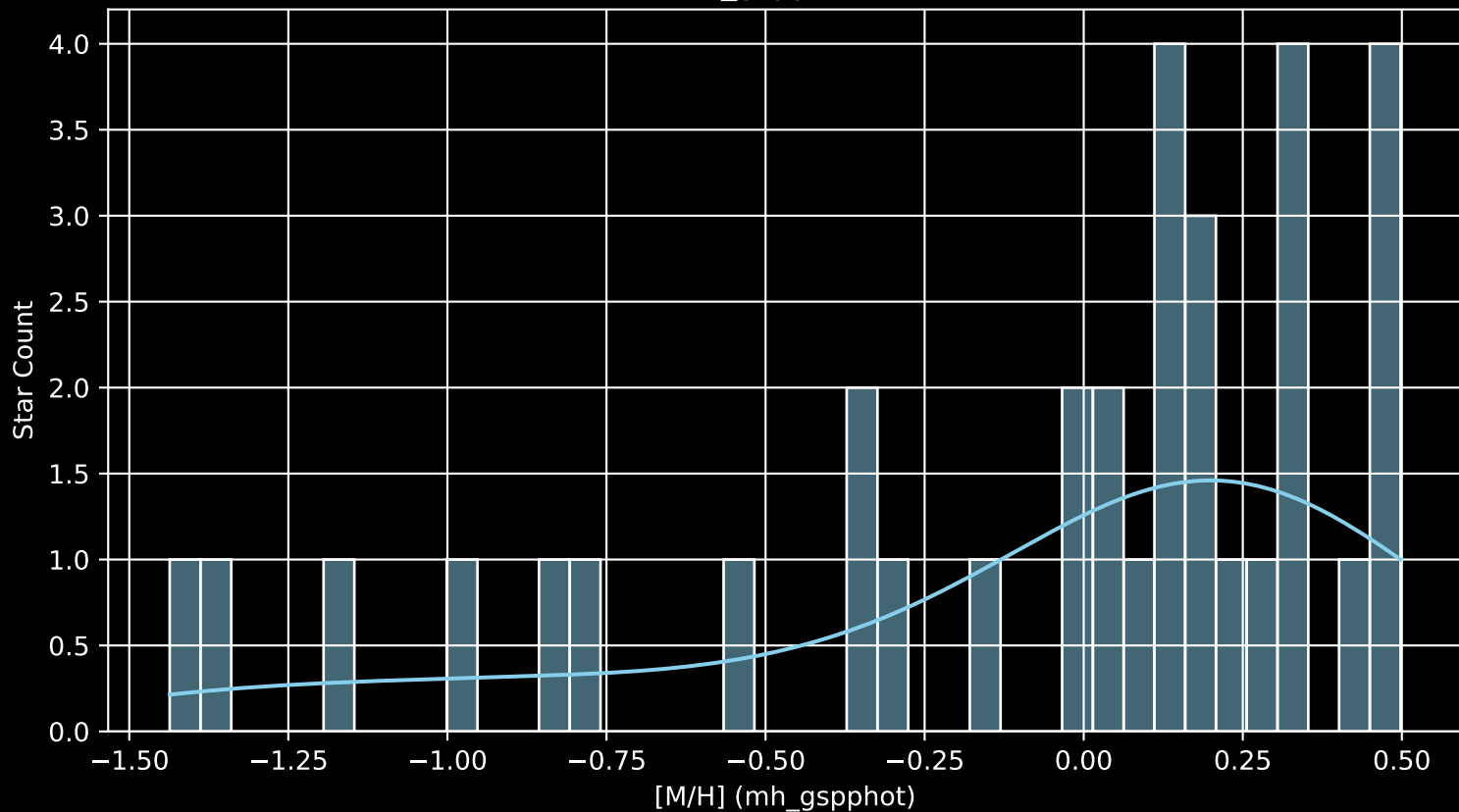
APOGEE DR17 Field: [280-32-O [M/H] (mh_gspphot) (n= 34)
